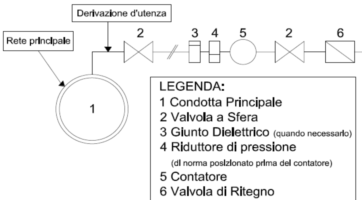
SCHEMA ALLACCIAMENTO ALL'ACQUEDOTTO COMUNALE (N.B. I vari componenti devono essere installati secondo l'ordine in figura)
